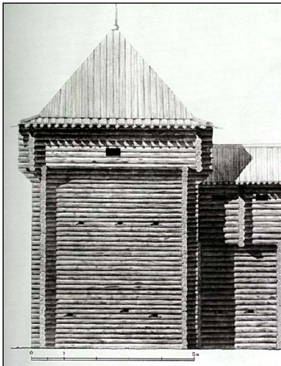
Рис. 6. Вариант башни Обоянского острога (из кн.: Крадин Н. П. Русское деревянное оборонное зодчество. М., 1988. Рис. 103–106)
