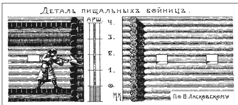
Рис. 7. Пищальные бойницы
