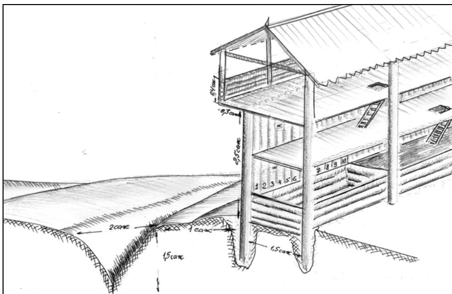
Рис. 5. Вариант конструкции стены Обоянского острога
